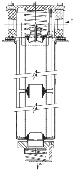
Dempster® Filter Assembly
